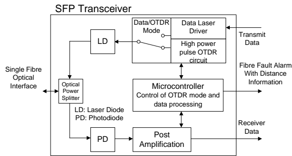
Fig. 2: SFP OTDR Module block diagram
